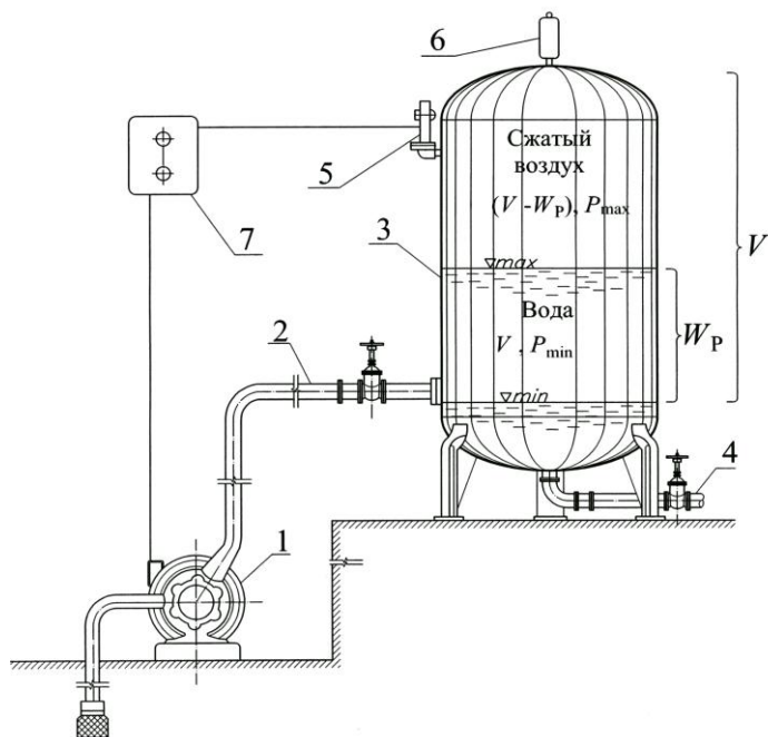
Рис. 1. Схема пневматической установки
