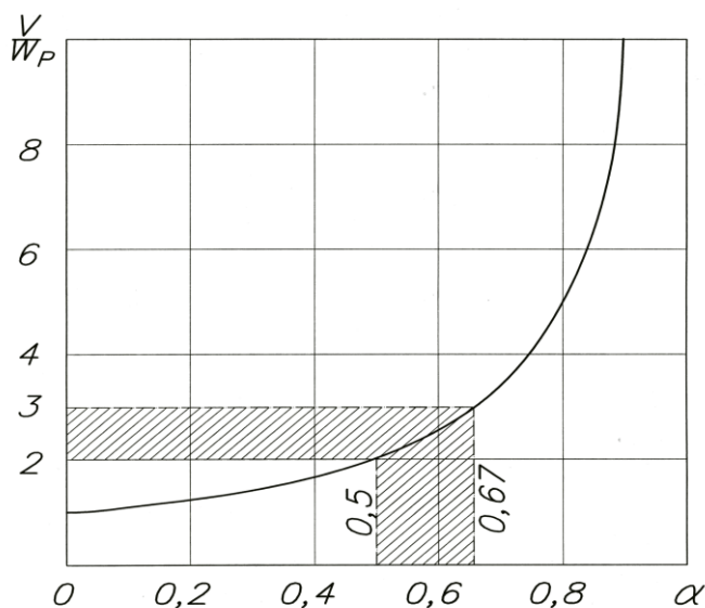
Рис. 3. График зависимости отношения V к W_p от \alpha
