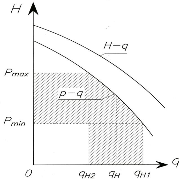
Рис. 2. работа насоса с котлом
